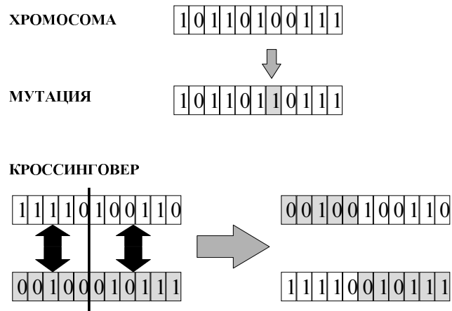
Рисунок 4. Представление искомого решения в виде битовой строки - хромосомы (вверху). Операции мутации и кроссинговера (внизу)
